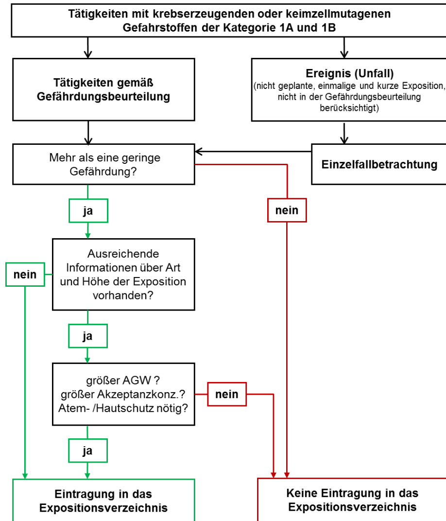
Vereinfachtes Ablaufschema, nach TRGS 410
